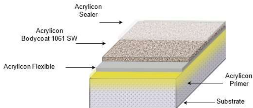
Figur 1: AcryliCon Décor System, opbygning
