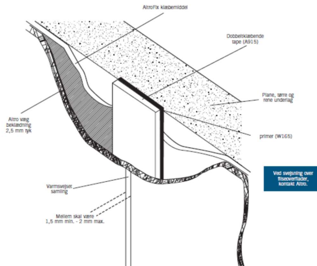
Figur 1 Princip skitse
