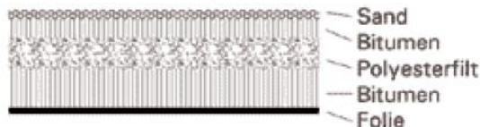
Figur 3 Opbygning af PTM DuraFlex
